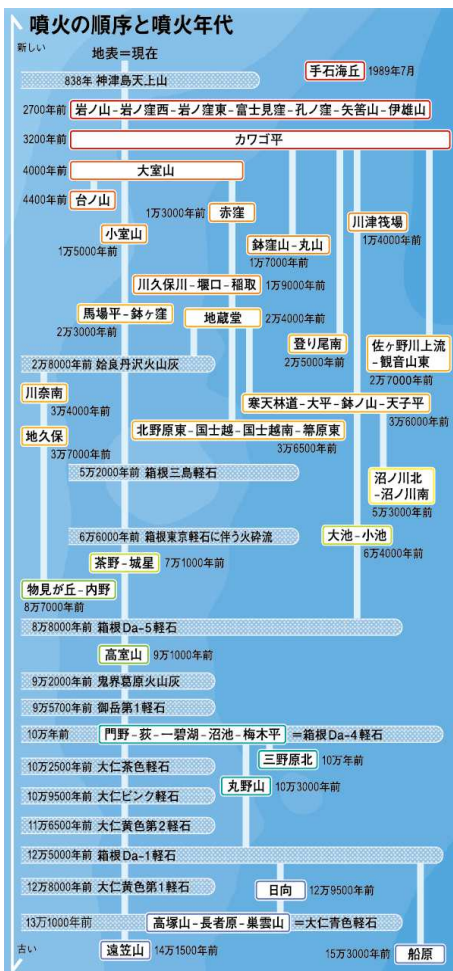
図1 伊豆東部火山群(陸域部分)の噴火順序と噴火年代(年代が判明しているもののみ)
