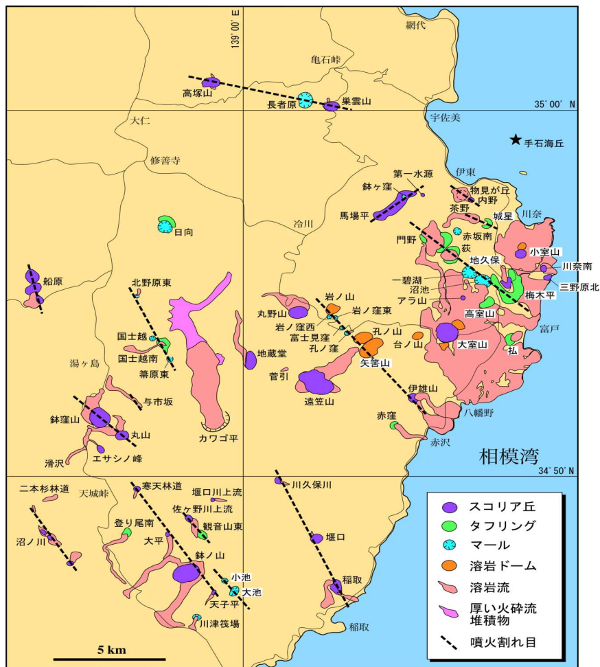
図2 伊豆東部火山群の分布図(陸域部分)
