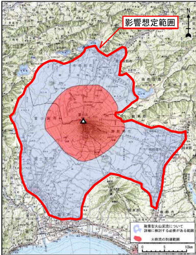
図4 融雪型火山泥流の影響想定範囲
