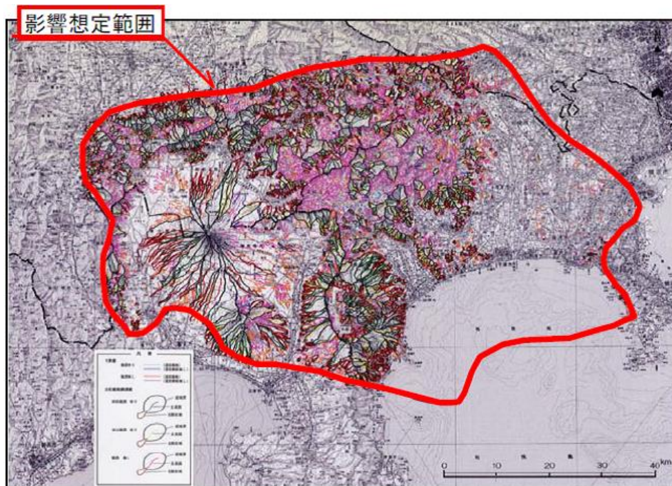
図5 降灰後土石流の影響想定範囲
