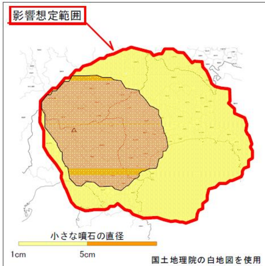
図3 小さな噴石の影響想定範囲
