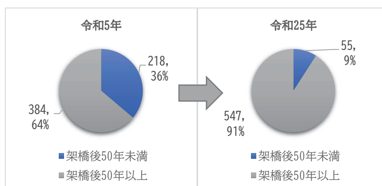
図1 架橋後50年以上の橋梁数
