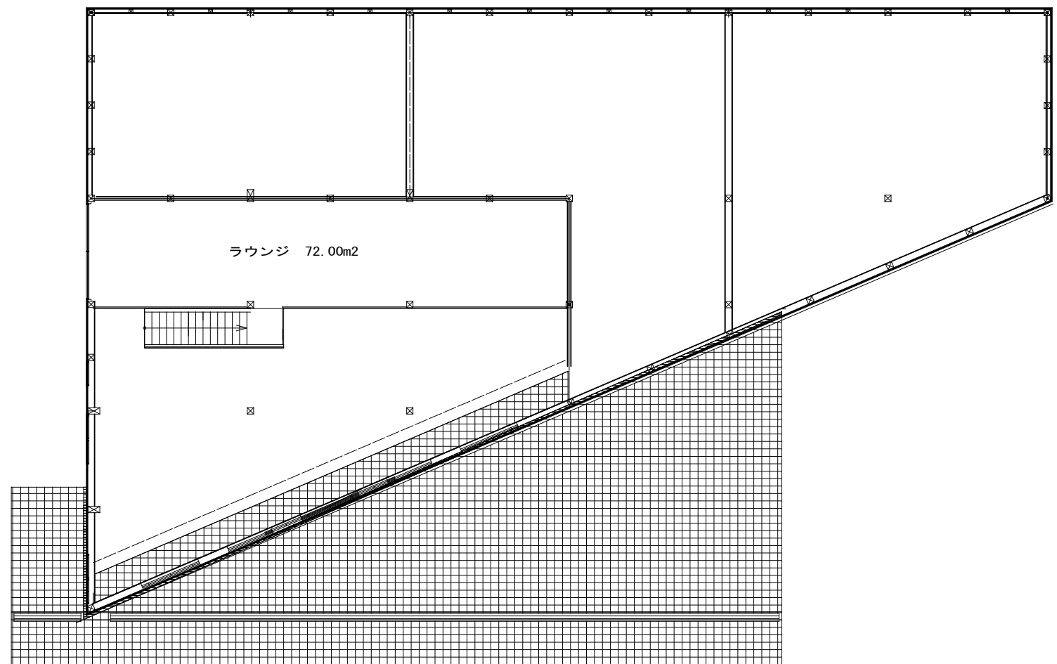
2階平面図
