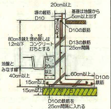
地盤の高低差が80cmを越え1.2m以下の場合の基礎
